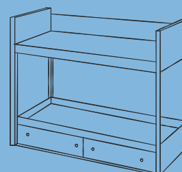
..... LETTO A CASTELLO CON MONTANTI 9723
